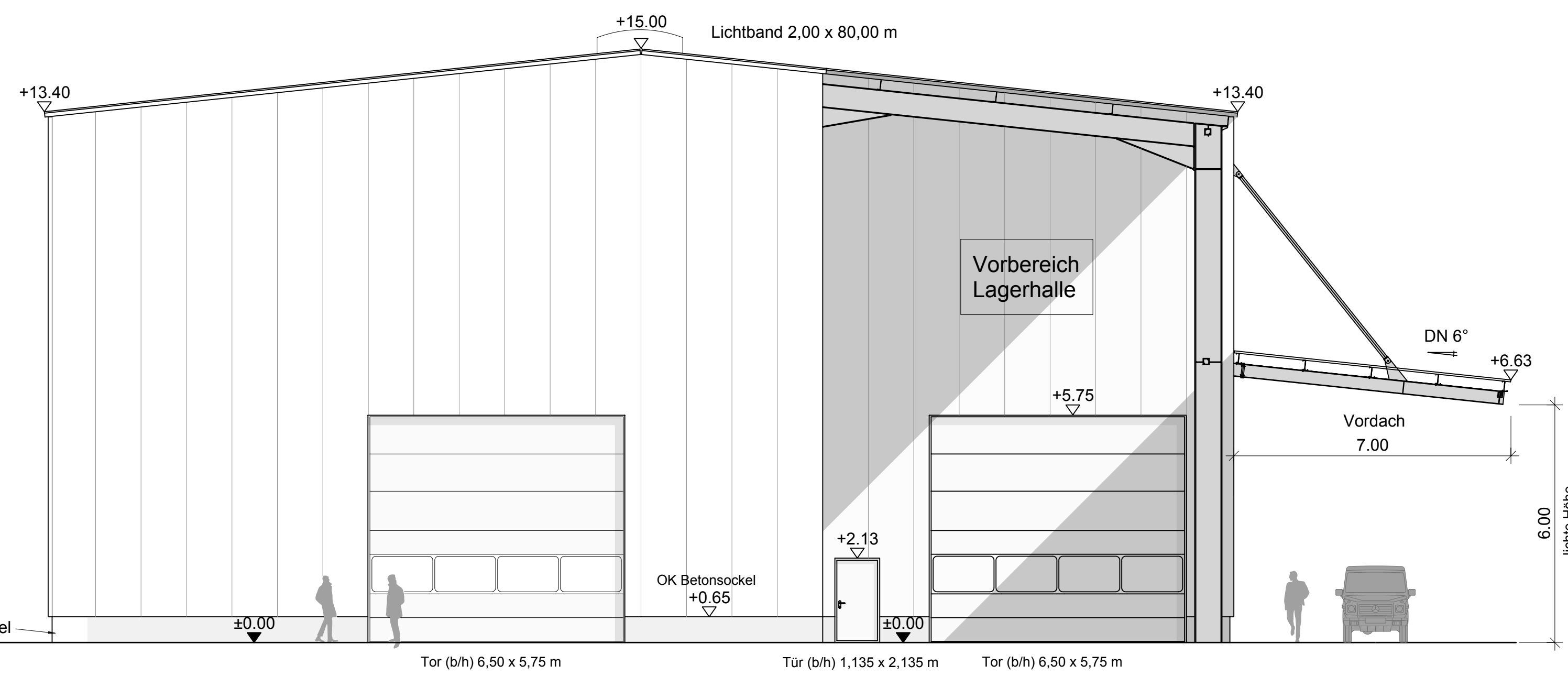
Ansicht Ost
