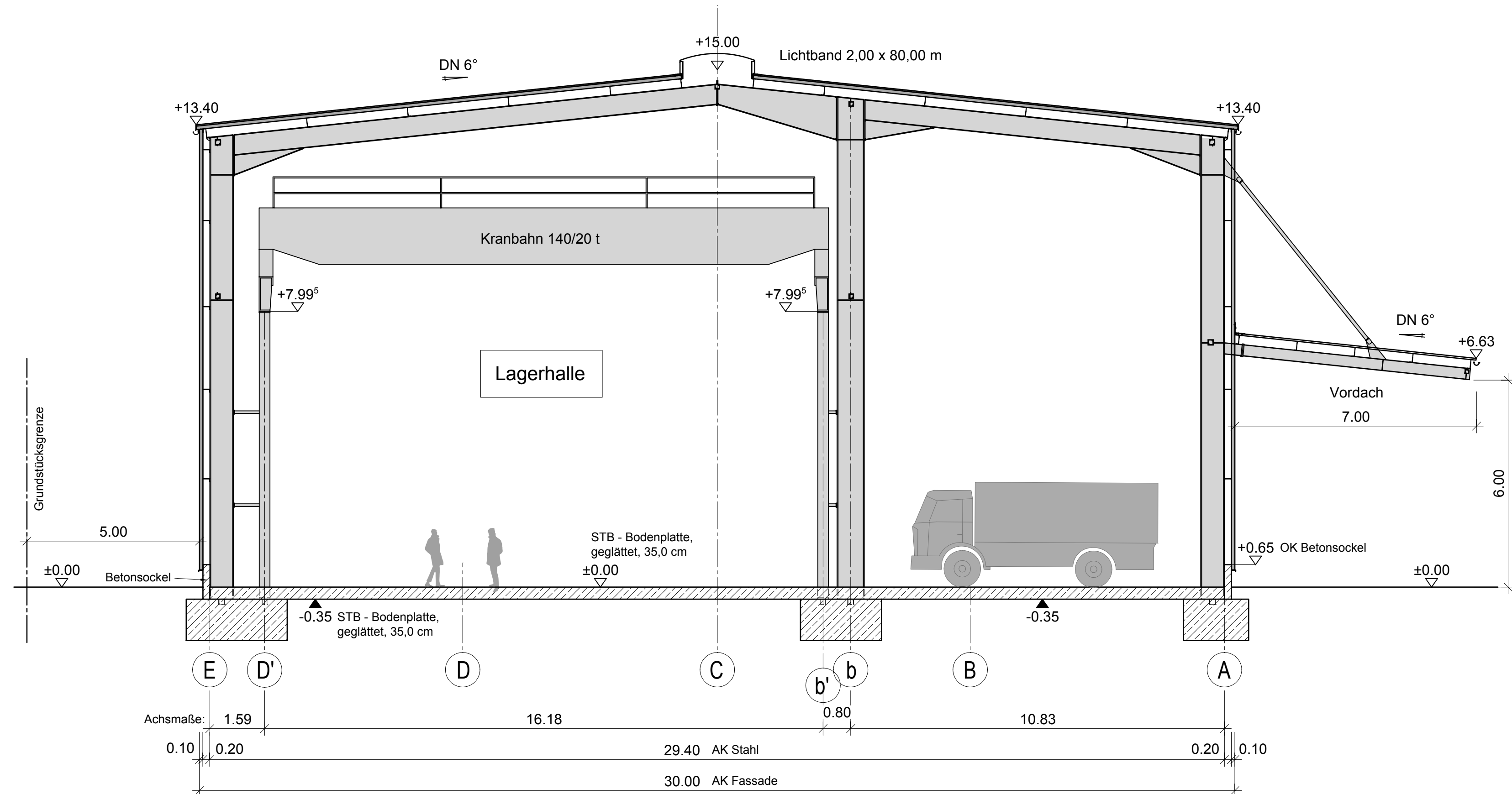
Schnitt A-A (Achse 5-10)
