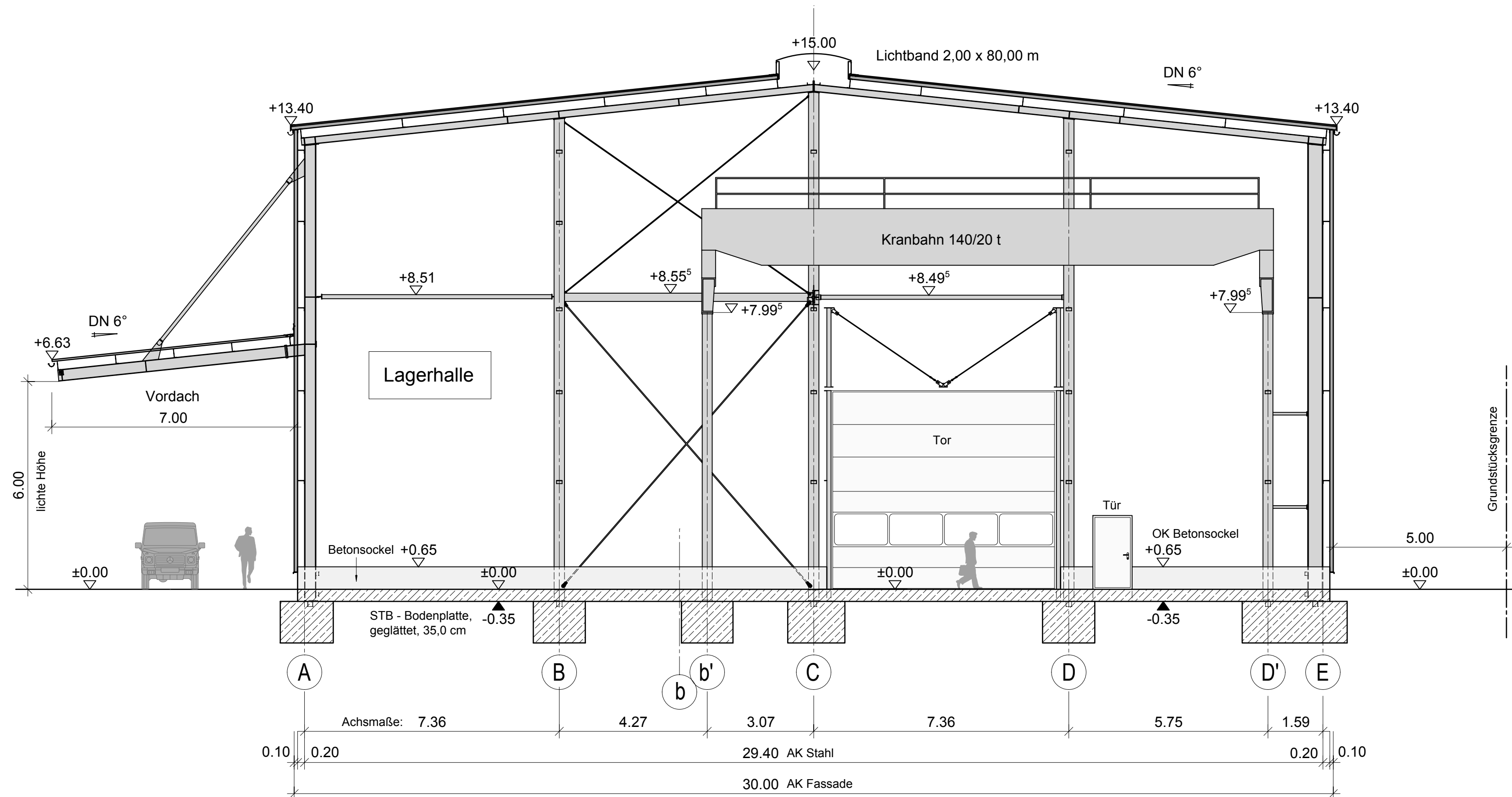
Schnitt B-B (= Achse 11)
